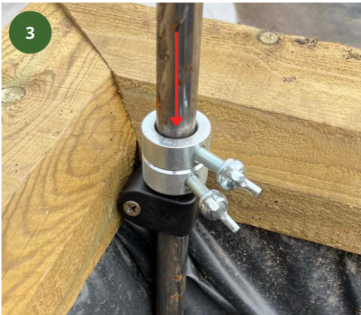
Skub pælen gennem beslaget – før pælen ned gennem beslaget, og påsæt BEGGE ringe.
