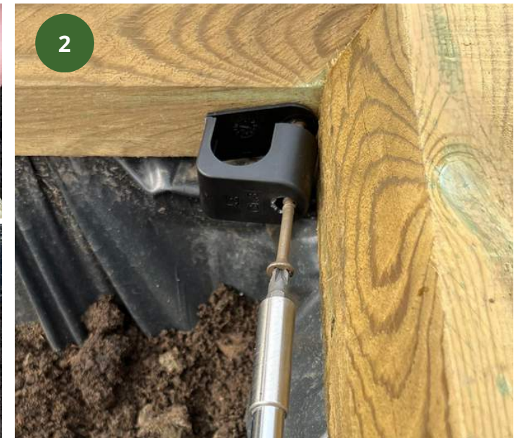
Skru beslaget på afslutningslaget – fastgør beslaget indvendigt i hjørnet på afslutningslaget.
